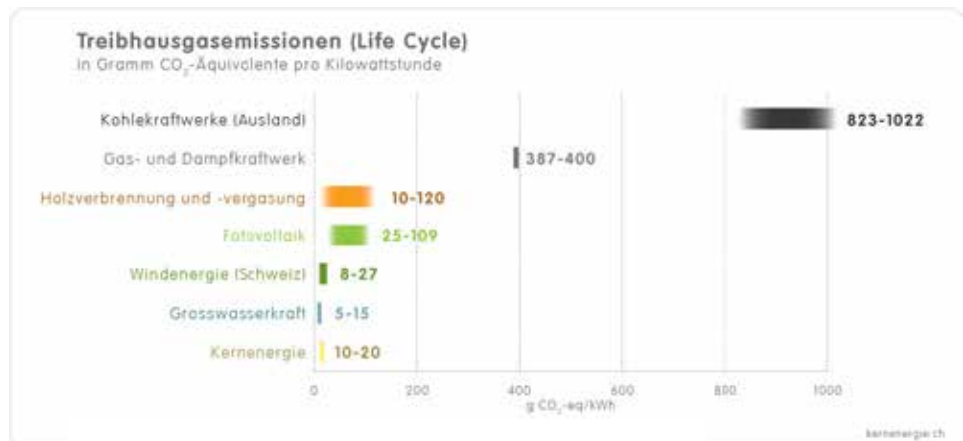
Grafik 2 Treibhausgasemissionen nach Stromproduktions- technologie in der Schweiz, BFE 2019
